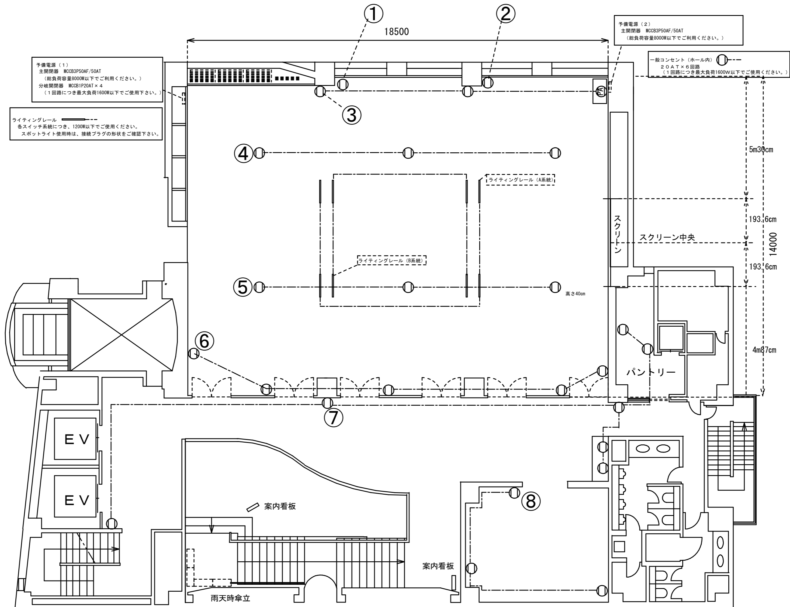
銀座フェニックスプラザ 2階ホール図面
